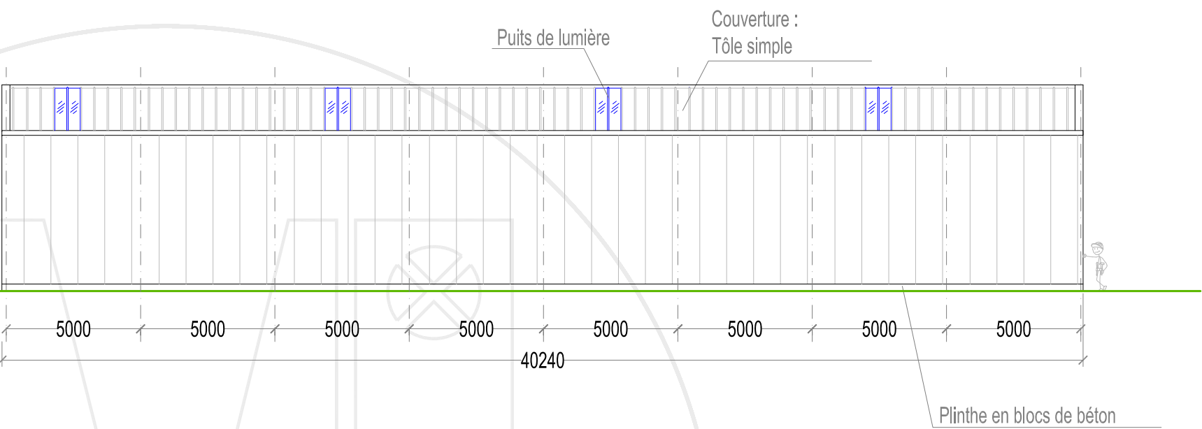
Toiture
